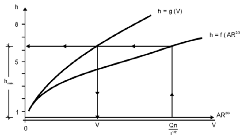
Figura 35 - Gráficos de h = f(AR^{2/3}) e h = g(V)
