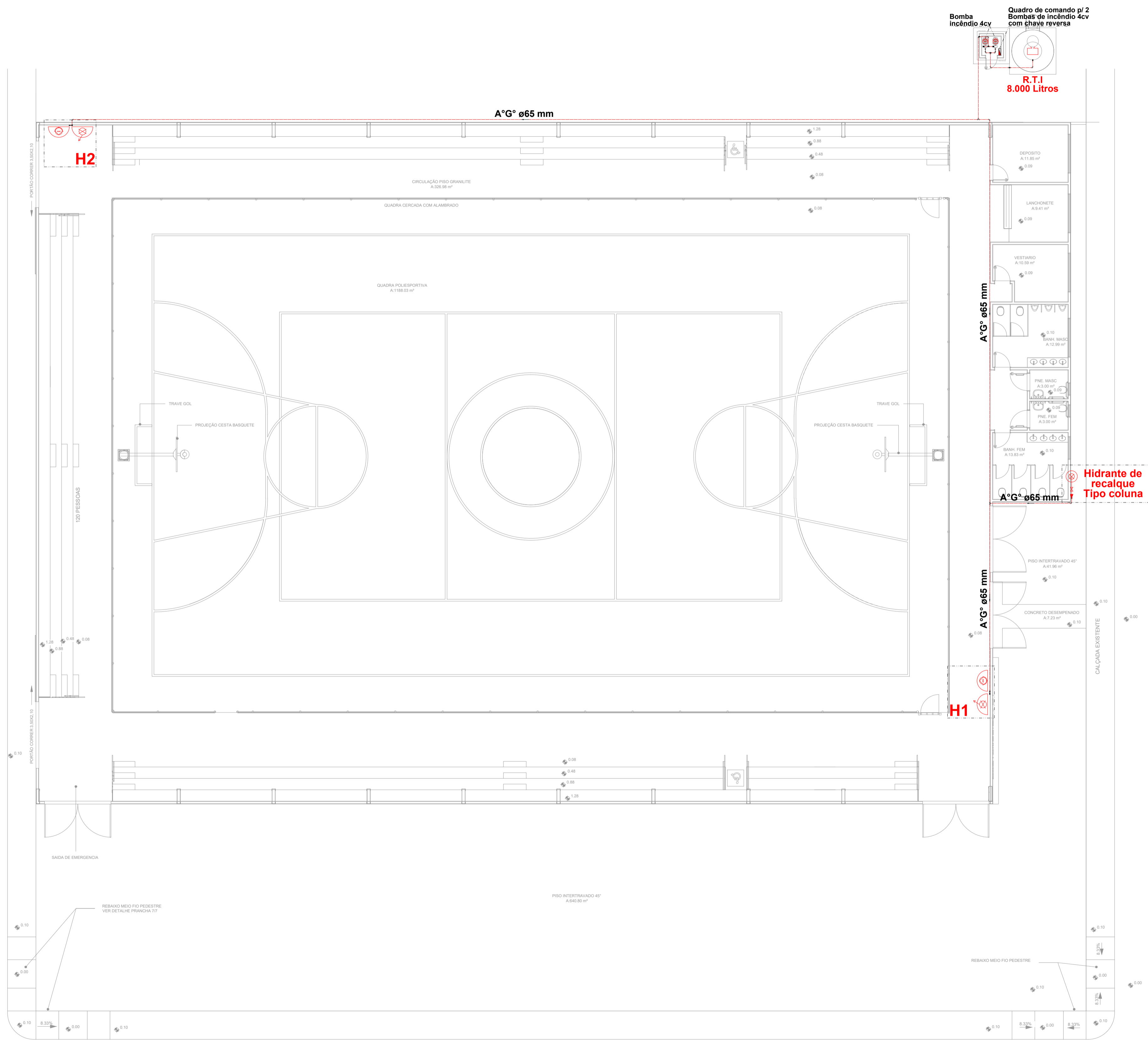
1 Planta baixa - Rede de hidrantes ESCALA: 1:125
